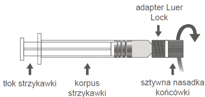
Rycina A: Strzykawka z końcówką Luer Lock ze sztywną nasadką końcówki, ang. Rigid Tip Cap:
