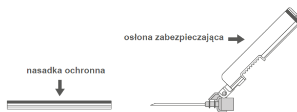
Rycina C: Elementy osłony zabezpieczającej igłę (przygotowane do użycia)
